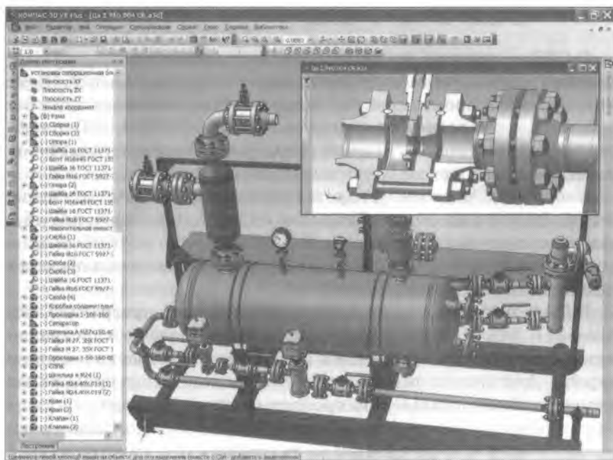
Рис. 8.2. Трехмерная модель сепарационной установки
