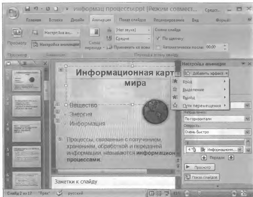
Рис. 5.11. Настройка анимации
