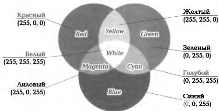
Рис. 7.1. RGB-модель цветопередачи
