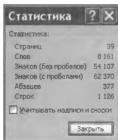
Рис. 3.29. Окно Статистика
