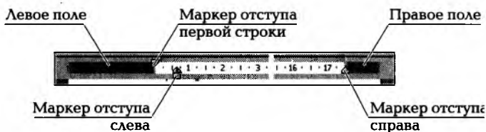
Рис. 3.3. Горизонтальная линейка
