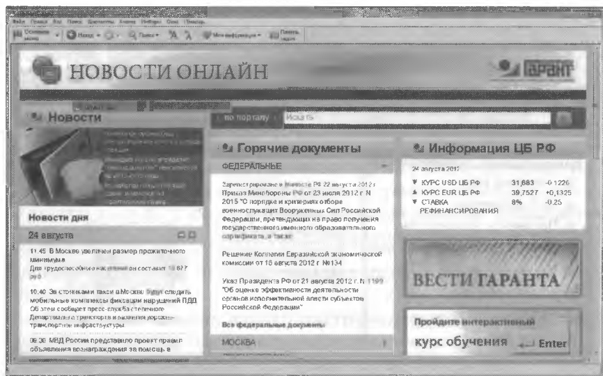
Рис. 9.9. Новости онлайн
