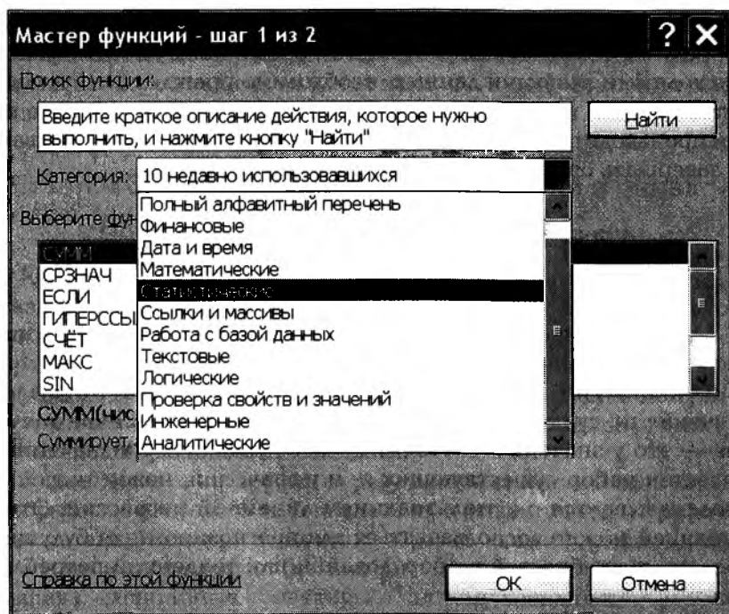
Рис. 4.7. Мастер функций
