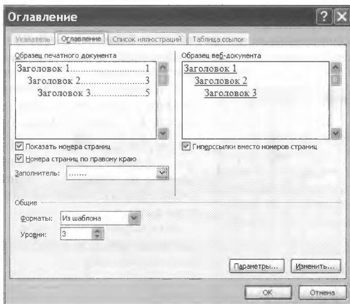
Рис. 3.17. Создание оглавления
